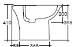
BIDET BIDET
